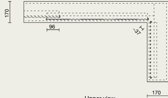
Upper view Vista dall'alto
